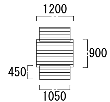
テーブル 2台 ベンチ 4台 (W1200 × D900 × H700) (W1050 × D450 × H415)
